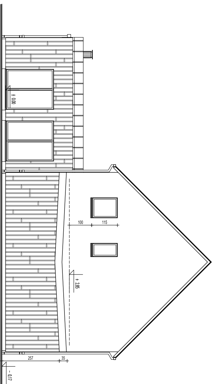
Façade SUD
